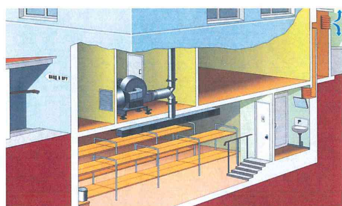
Противорадиационное укрытие
